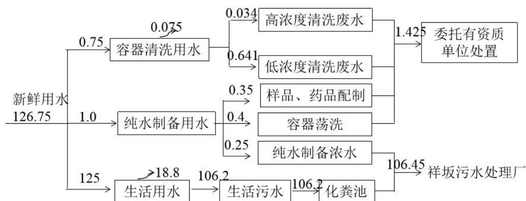
图 2.1-1 本项目水平衡图 (t/a)
