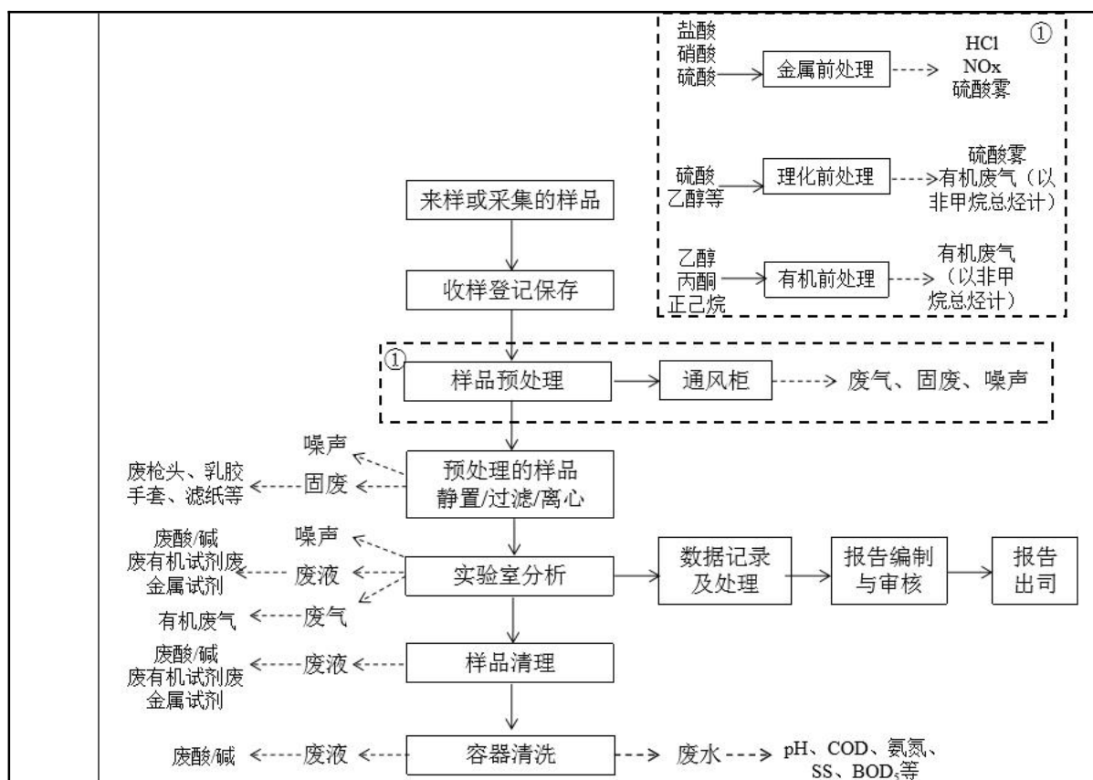
图 2.2-2 检测实验室工艺流程及产排污环节示意图
