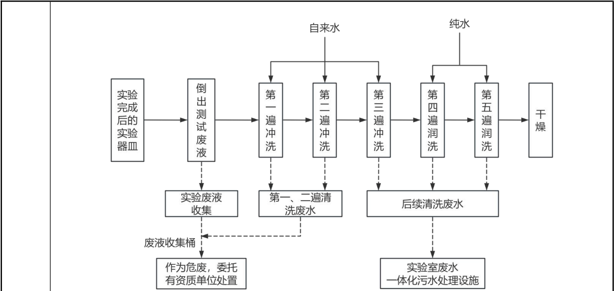
图 2.8-5 实验器皿清洗流程及产污环节示意图
