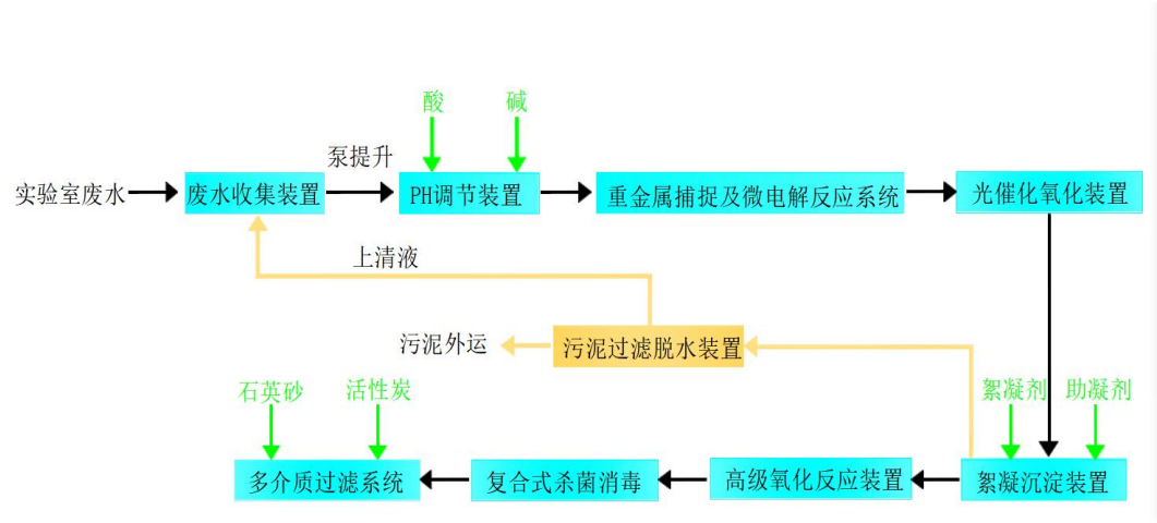
图 4.2-1 一体化污水处理设施工艺
